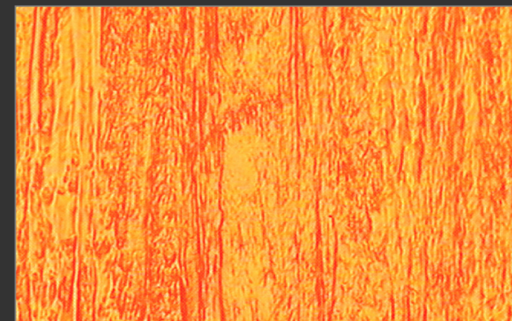
大晶銅 / 縱 100 倍 / 晶相
