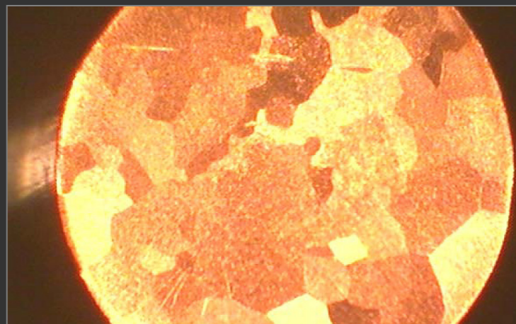
大晶銅 / 橫 15 倍 / 晶相
